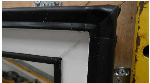
Fot.6 Złożenie blach osłonowych w narożu skrzydła
