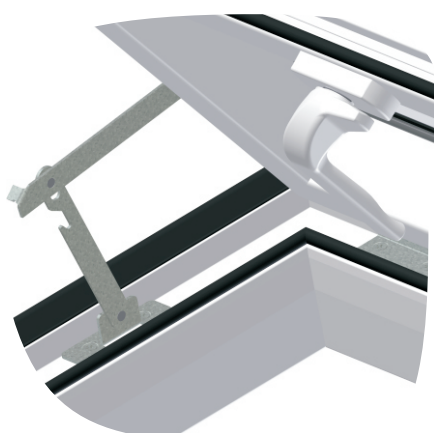
4a. Pozycja pośrednia w trakcie otwierania: -widok ogranicznika otwarcia/zamknięcia.
