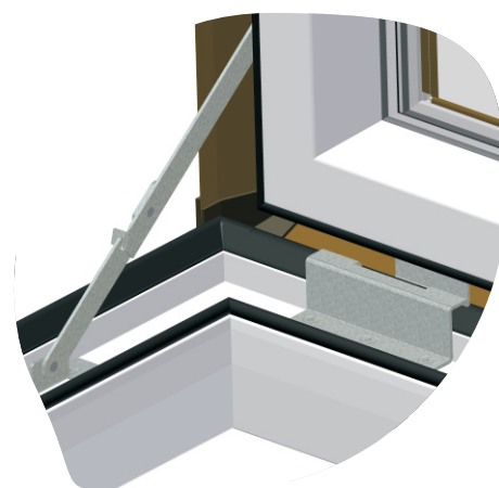
4c. Zablokowany ogranicznik otwarcia/zamknięcia-pozycja zahamowana,skrzydło otwarte o 90°.
