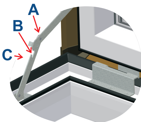
4b. Aby ustawić skrzydło w pozycji zahamowanej otwartej należy umieścić część skrzydłową ogranicznika otwarcia/zamknięcia A w gnieździe B części ramowej ogranicznika C jak na rys. 4c.
