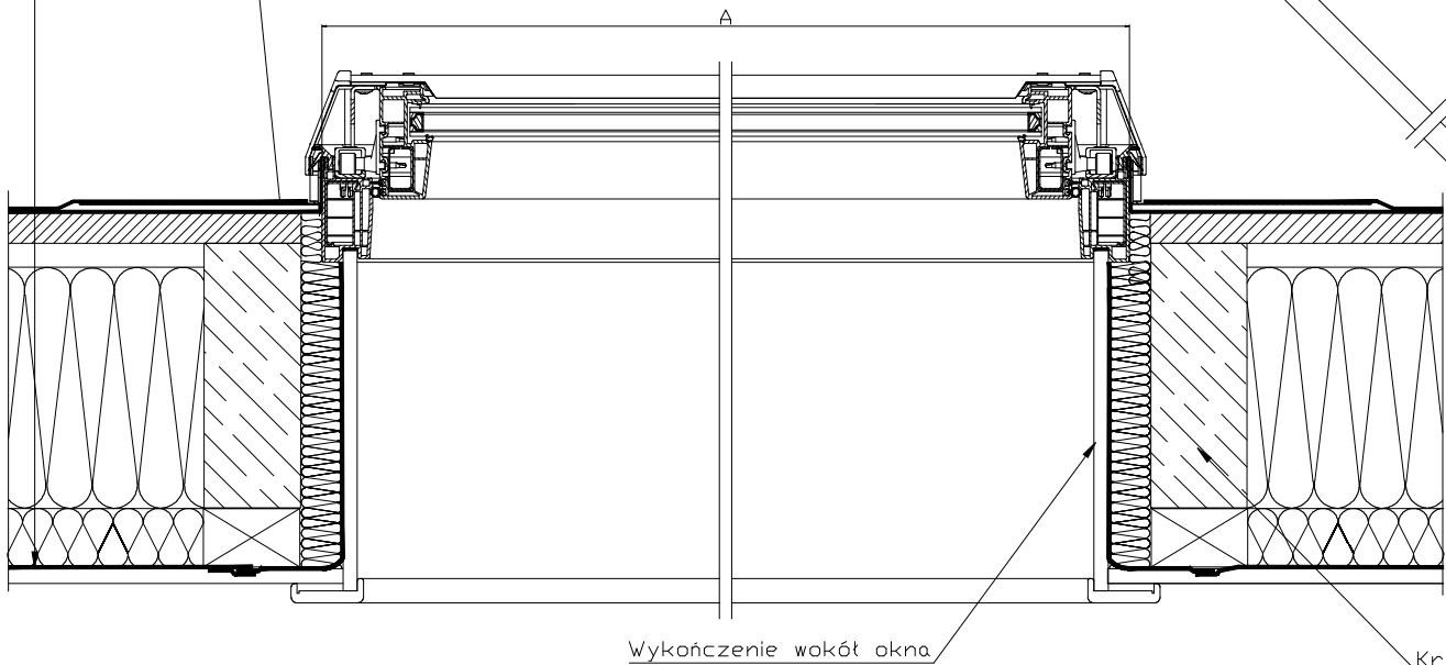
PRZEKRÓJ A-A
