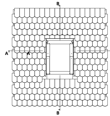
PRZEKRÓJ B-B
